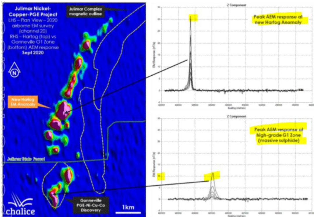
Figure 2. Hartog EM Anomaly Plan View – Airborne EM survey preliminary late-time response.
