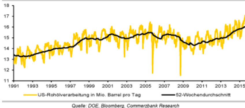
GRAFIK DES TAGES: US-Rohölverarbeitung liegt auf außerordentlich hohem Niveau
