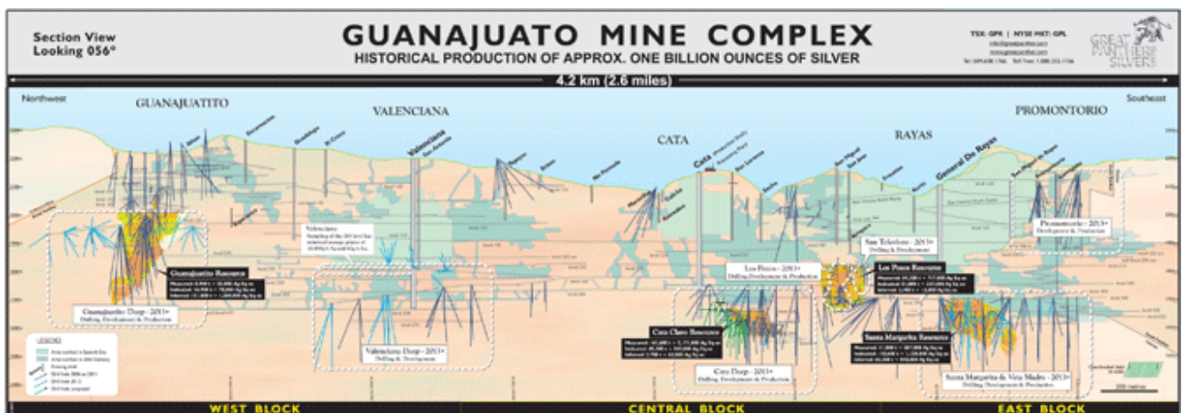
Schnittbild des Guanajuato Minenkomplexes (zur Vergrößerung klicken sie bitte hier (PDF))
