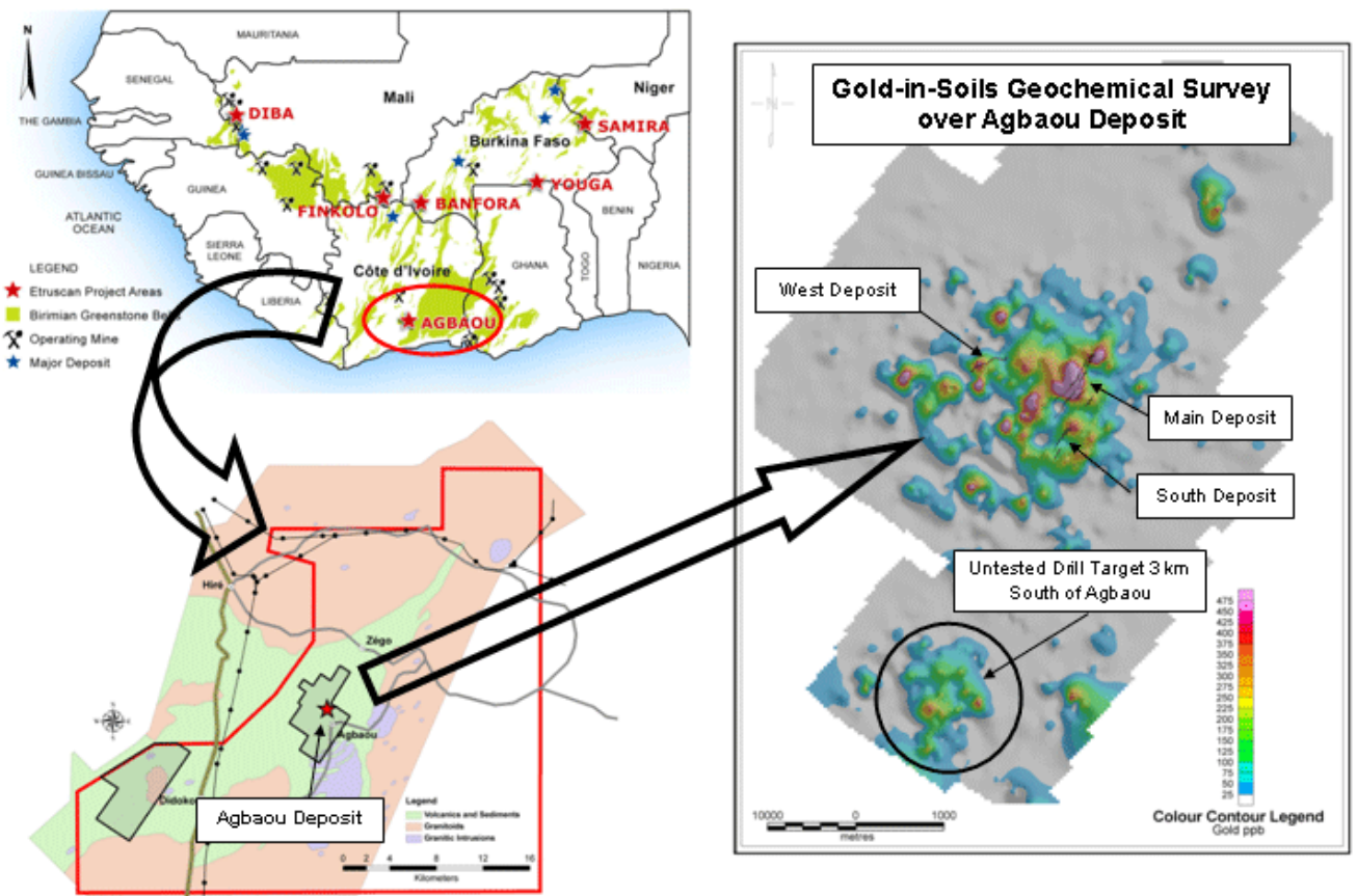
Darstellung 2 - 6. Dezember 2007, Lage der Explorationsbohrungen für Tests auf Satellitenlagerstätten der Agbaou Konzession, Elfenbeinküste
